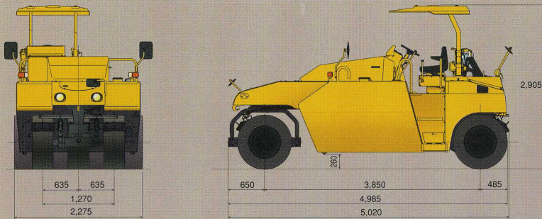
外觀図 単位：mm
