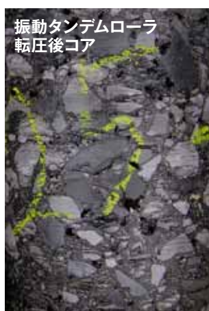
図5 厚層締固め後のコア比較（最大粒径37mm、仕上厚25cm）
