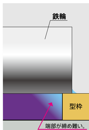
図3 ブリッジング現象の解消
