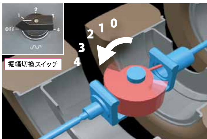
可変振幅振動機構のイメージ図
