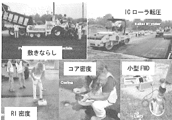
写真一1 試験施工と管理機器による測定
